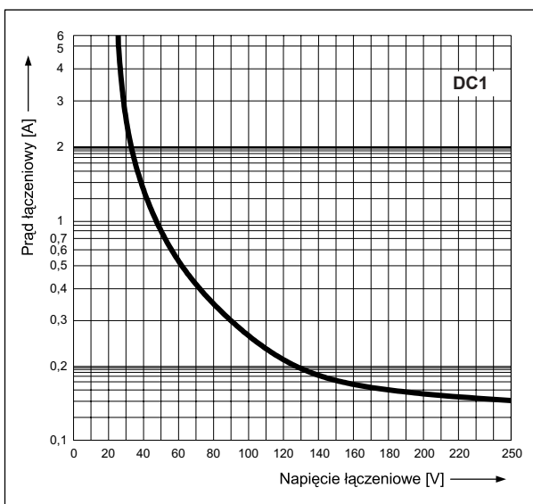
Maksymalna zdolność łączeniowa dla prądu stałego. Obciążenie rezystancyjne Wykres 3
