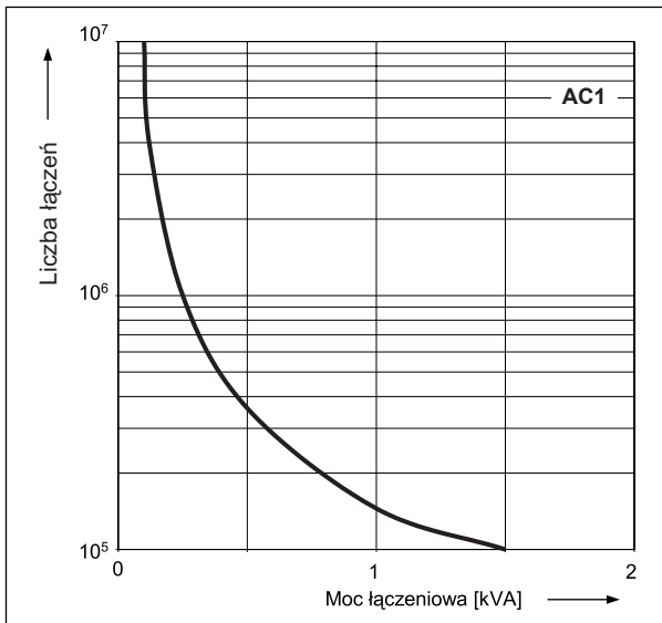
Trwałość łączeniowa w funkcji mocy obciążenia. Obwód bezindukcyjny. Maksymalna częstota łączy przy obciążeniu znamionowym Wykres 1
