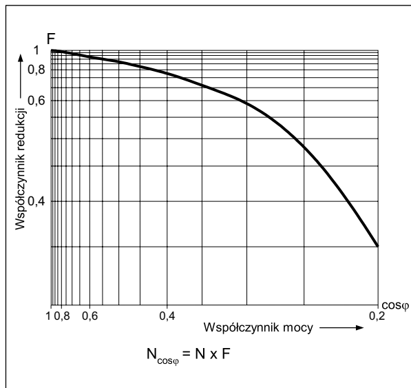
Współczynnik redukcji łączeniowej dla indukcyjnych obciążeń prądu przemiennego Wykres 2
