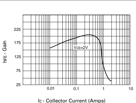
h_{FE} v I_C
