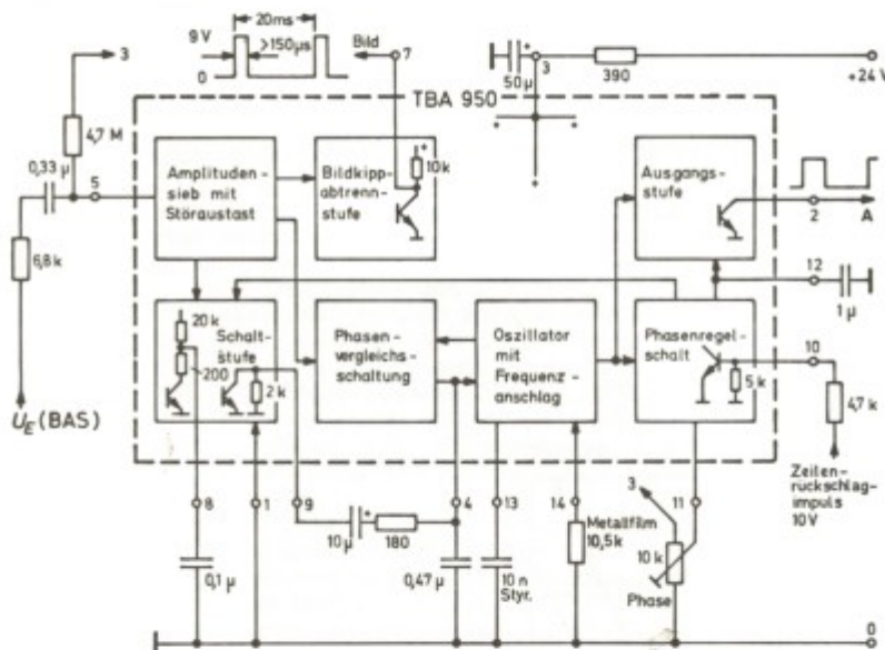
Bild 1: Blockschaltbild des TBA 950 und Meßschaltung für die Kennwerte.
