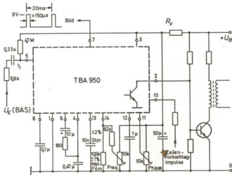
Bild 5: Betriebsschaltung des TBA 950, Alternativvorschlag zur Frequenz-einstellung
