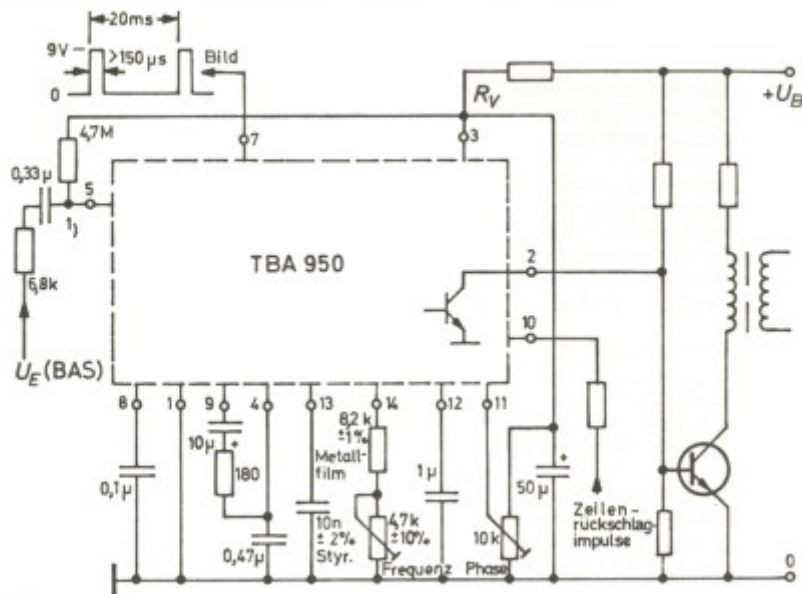
Bild 4: Betriebsschaltung des TBA 950
