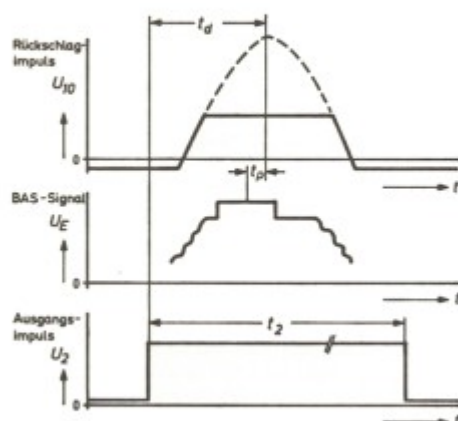
Bild 3: Phasenbeziehungen beim TBA 950. Der begrenzte Zeilenrückschlagimpuls muß den Zeilenimpuls des BAS-Signals beidseitig überlappen.
