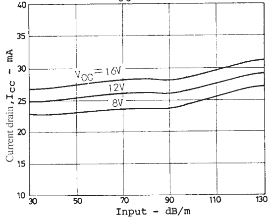
I_{CC} - Input
